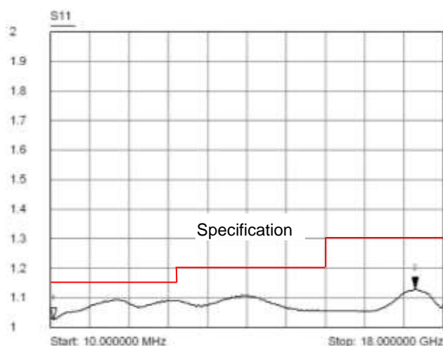
TC18-01-03-1000 的典型 S11 指标:
