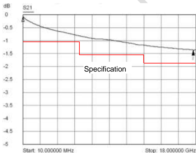
TC18-01-03-1000 的典型 S21 指标:
